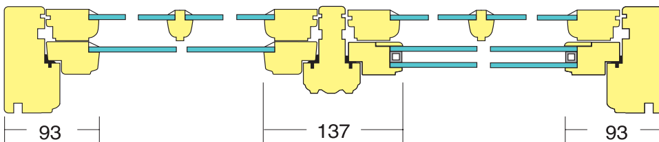
Snitt av 2 rams vindu, 1+1 lag til venstre og 1+2 lag til høyre.
