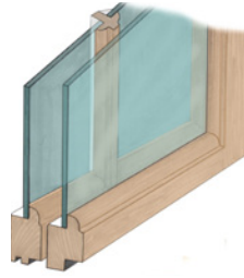
Snitt av kobla vindu med 1+1 lag glass.
