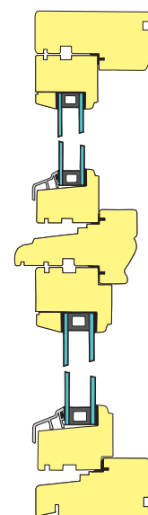
Snitt av losholtvindu.
