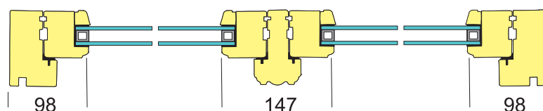
Snitt gjennom karm, ramme og post i et isolerglassvindu
