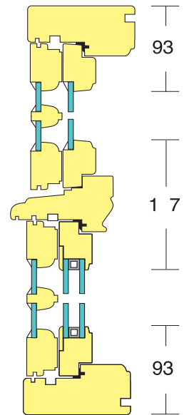
Snitt fra siden av losholtvindu. 1+1 lag oppe, 1+2 lag nede.
