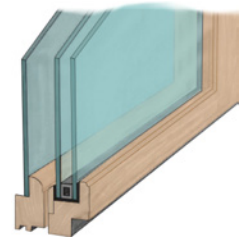
Snitt av kobla vindu med 1+2 lag glass.
